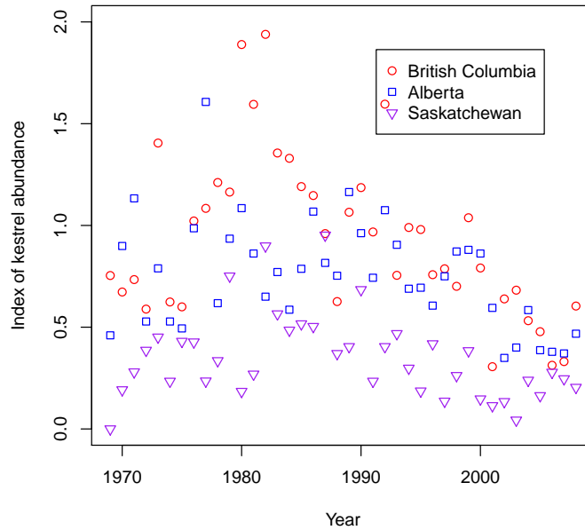
Fig. 15.3. The kestrel data.
