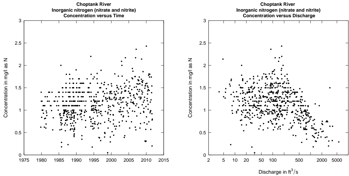
(a) plotConcTime(eList)
