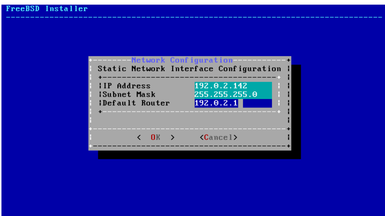
Рисунок 84. Статическая настройка IPv4 на сетевом интерфейсе
